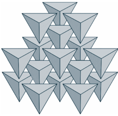
Die dichteste Tetraeder-Gitterpackung (aus: Conway & Torquato, PNAS 2006)
