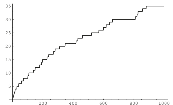
Anzahl der Primzahlzwillingspaare \leq n . Wie die Primzahlen selbst sind Primzahlzwillinge relativ häufig unter den kleinen Zahlen und werden allmählich seltener. Schon früh, etwa zwischen 670 und 800, gibt es weite Bereiche ohne ein einziges Zwillingspaar.
