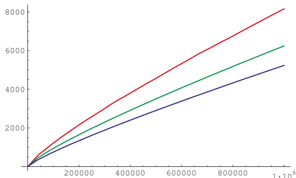
Die Anzahl der Primzahlzwillinge \pi_2(x) (hier bis zu einer Million; rot) übertrifft für jedes x die Werte der Schätzfunktionen li_2(x) (Integrallogarithmus; grün) und \frac{x}{(\log x)^2} (blau).
