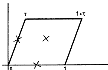
Fig. 3 Gitter mit Zweiteilungspunkten
