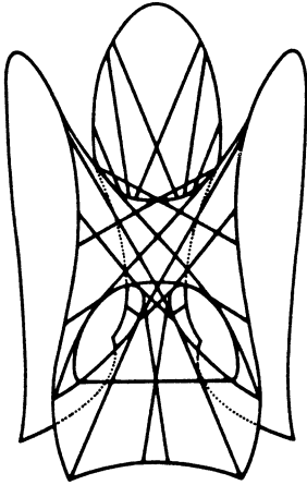
Fig. 4 Clebsche Diagonalfläche (nach P. Slodowy [SL], MPI Bonn)
