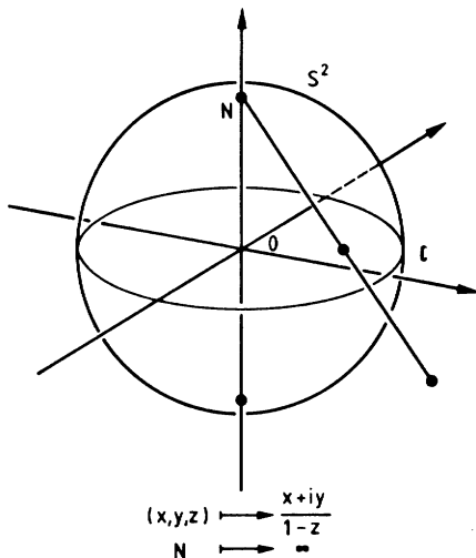
Fig. 2 Stereographische Projektion
