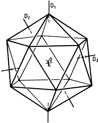
Fig. 1 Ikosaeder
